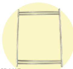
SB-V15 H800mm×W620mm× D620mm 支柱φ19 梁φ16 重量1.35kg
